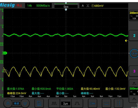
Noise VIN=52V,Io=1A 20MHz Bandwidth
